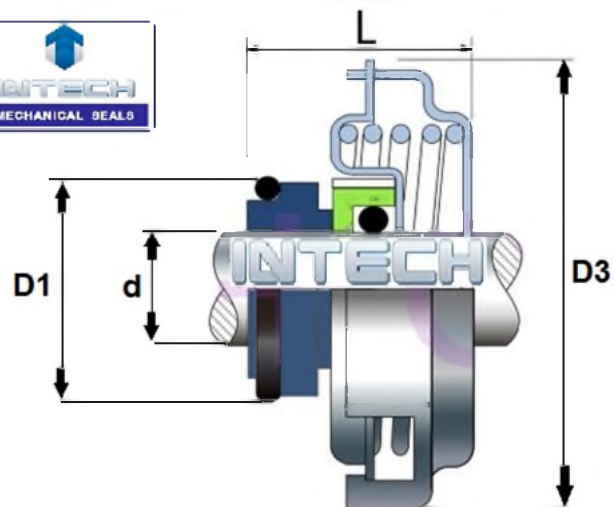
Rozměry mechanických ucpávek InTech GRCM do čerpadel Grundfos řady CM a CME
