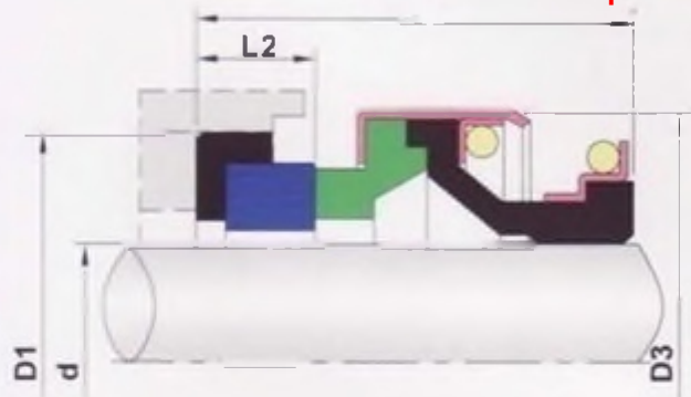
L = délka se stlačenou pružinou
